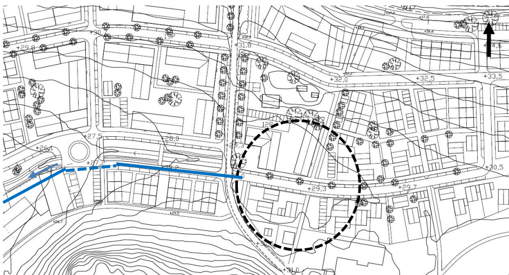
Figur 10. Preliminär höjdsättning av områdets centrala och södra delar. Område markerat samma som i figur 7. Dike blåmarkerat. (Arkitekterna Krook & Tjäder AB, 2017-04-11)
