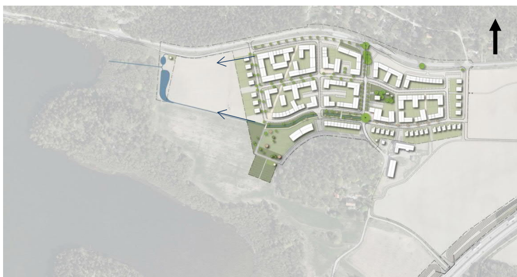
Figur 2. Illustrationsplan, tänkt bebyggelse och placering av dammar. Observera att bebyggelsen har ändrats något efter att figuren färdigställdes, se figur 3.
